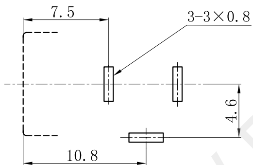
线路板开孔尺寸
